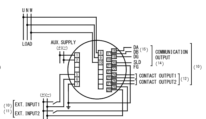
(10) Voltage input 1P3W
