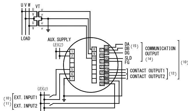
(9) Voltage input 3P3W
