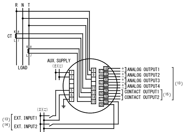
(2) 1 φ 3W
