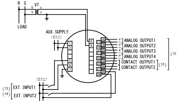
(11) Voltage input 1φ2W
