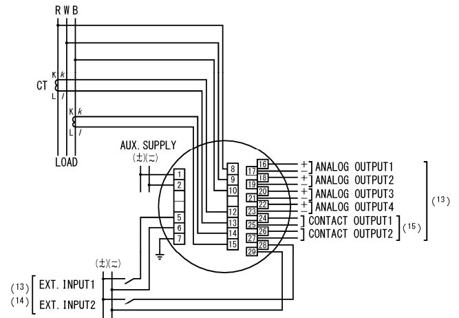
(2) 1P3W
