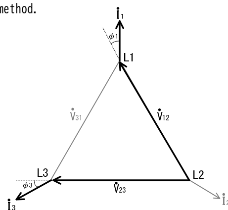
【Vector diagram (3P3W)】
