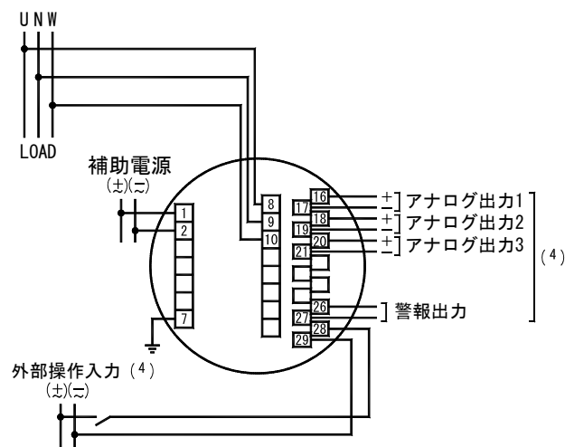
(2) 1φ3W, アナログ出力
