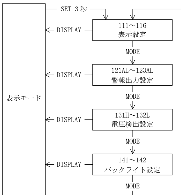
設定モード1
