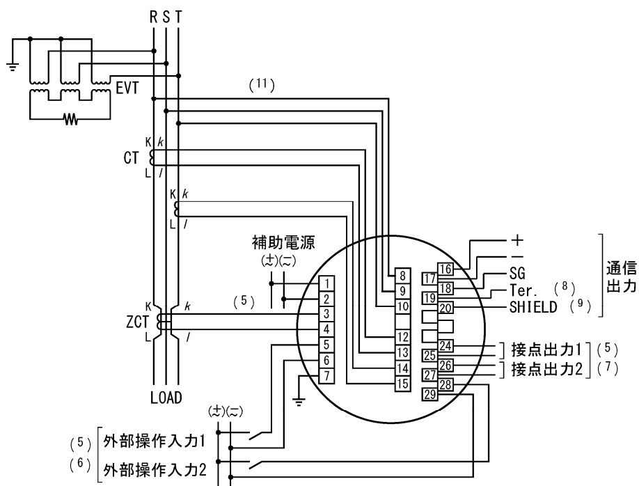
(4) 3 \phi 3W (S 相非接地)
