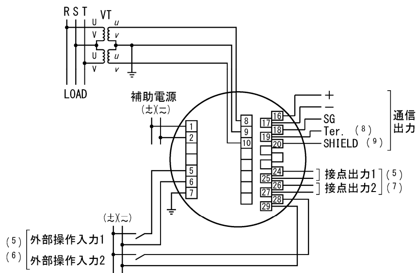
(9) 電圧入力 3 \phi 3W (2VT)
