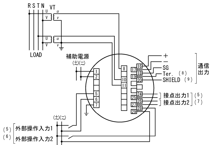
(10) 電圧入力 3 \phi 4W (2VT)
