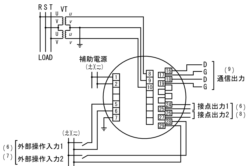
(9) 電圧入力 3φ3W (2VT)
