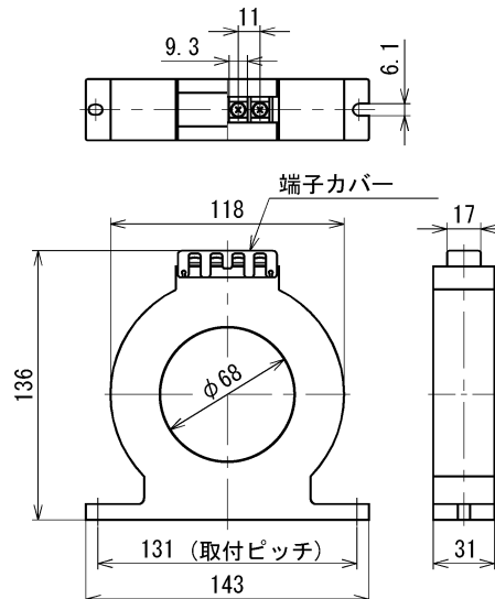
100A 屋外用 (OTG-LA30W)
