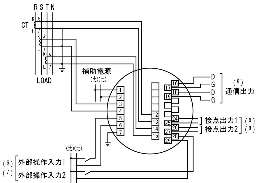
(16) 電流入力 3 \phi 4W (3CT)
