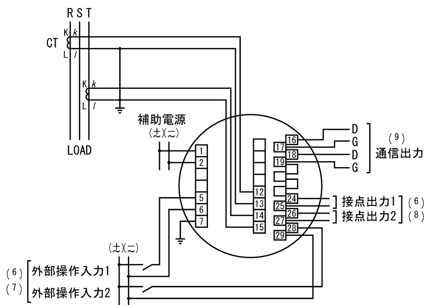
(14) 電流入力 3 φ 3W (2CT)
