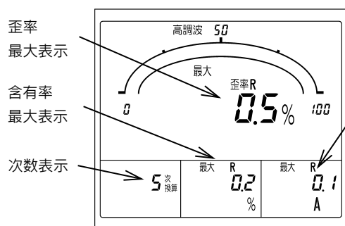
高調波電流最大表示
