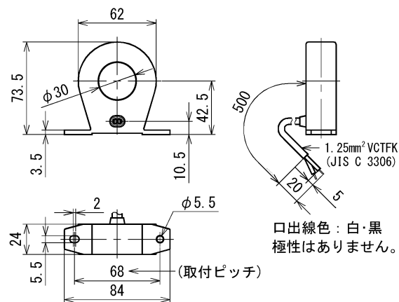
100A 屋外用 (OTG-LA30W)
