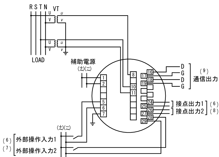
(10) 電圧入力 3φ4W (2VT)
