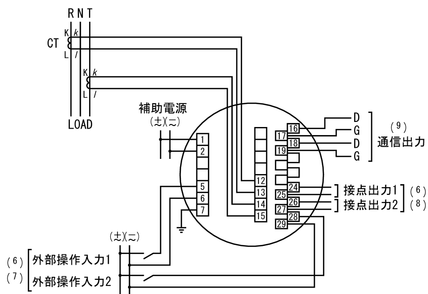
(13) 電流入力 1 φ 3W
