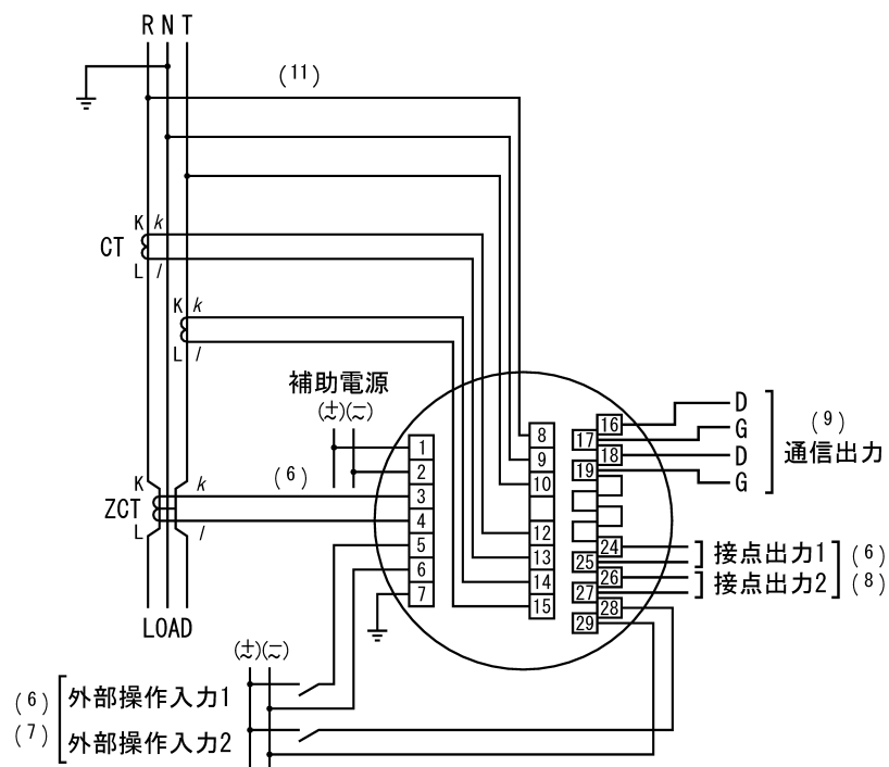
(2) 1 \phi 3W (N 相接地)
