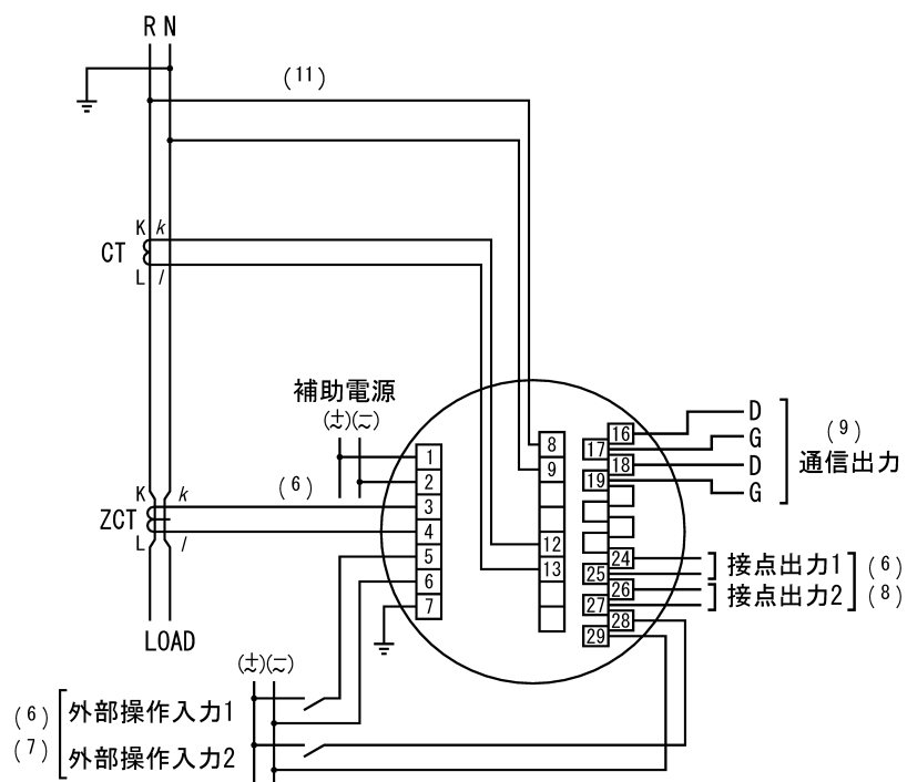
(1) 1 \phi 2W (N 相接地)
