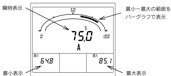
一般計測最大/最小表示
