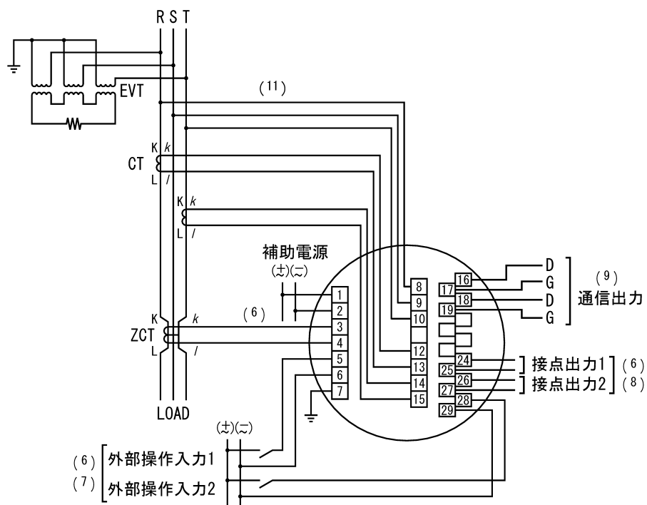
(4) 3 \phi 3W (S 相非接地)
