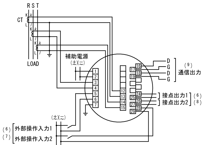
(15) 電流入力 3 \phi 3W (3CT)
