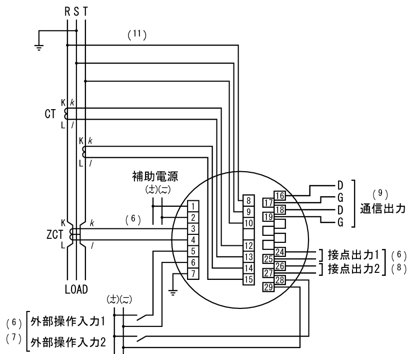
(3) 3 \phi 3W (S 相接地)
