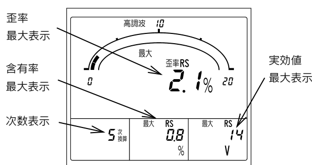
高調波電圧最大表示
