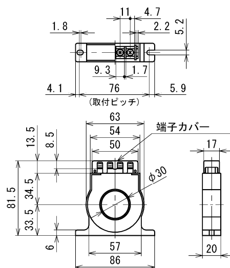
400A (OTG-LA68)
