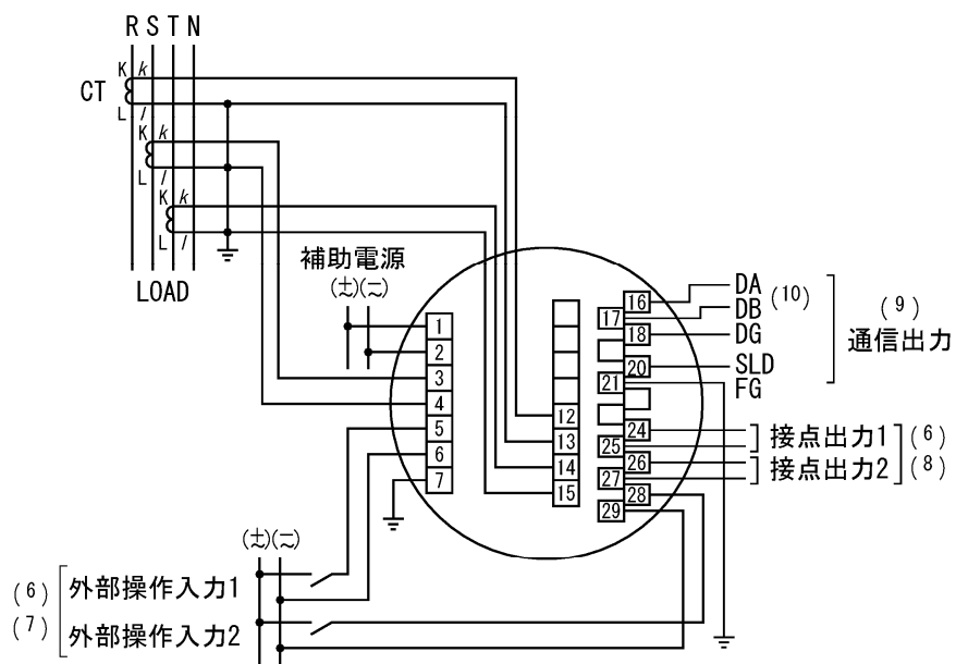
(16) 電流入力 3 \phi 4W (3CT)
