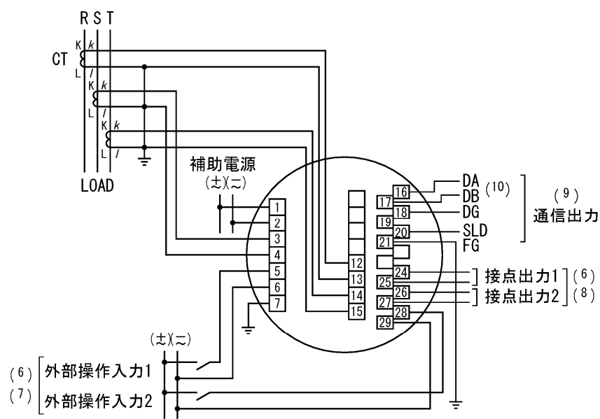
(15) 電流入力 3 \phi 3W (3CT)
