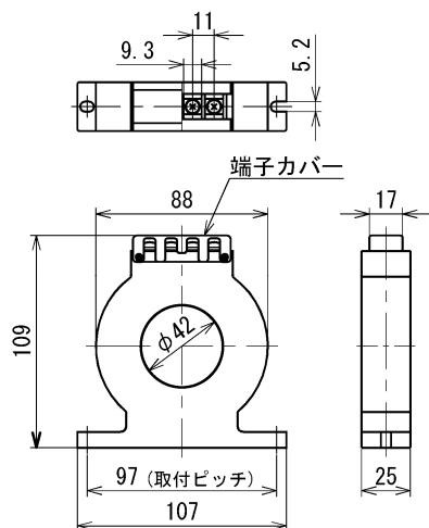
200A (OTG-LA42)
