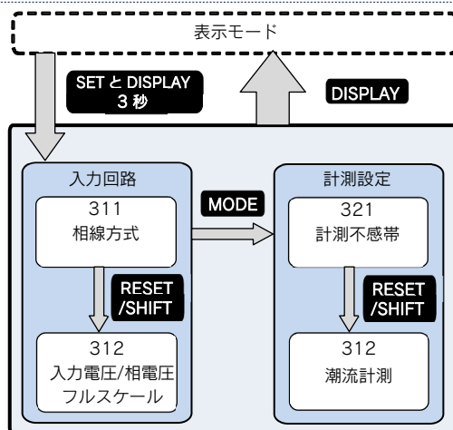
3φ3W/1φ3W/1φ2W の場合
