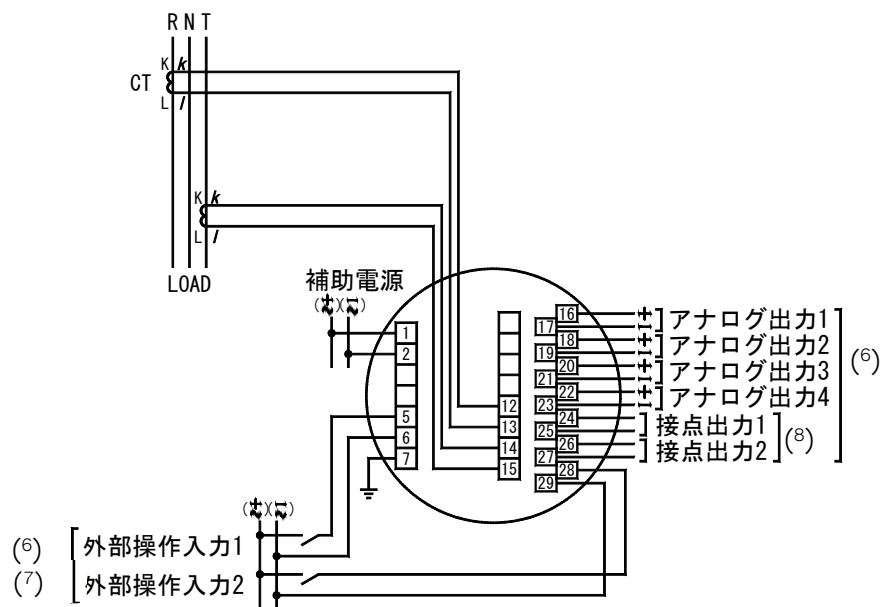
(13) 電流入力 1 \phi 3W
