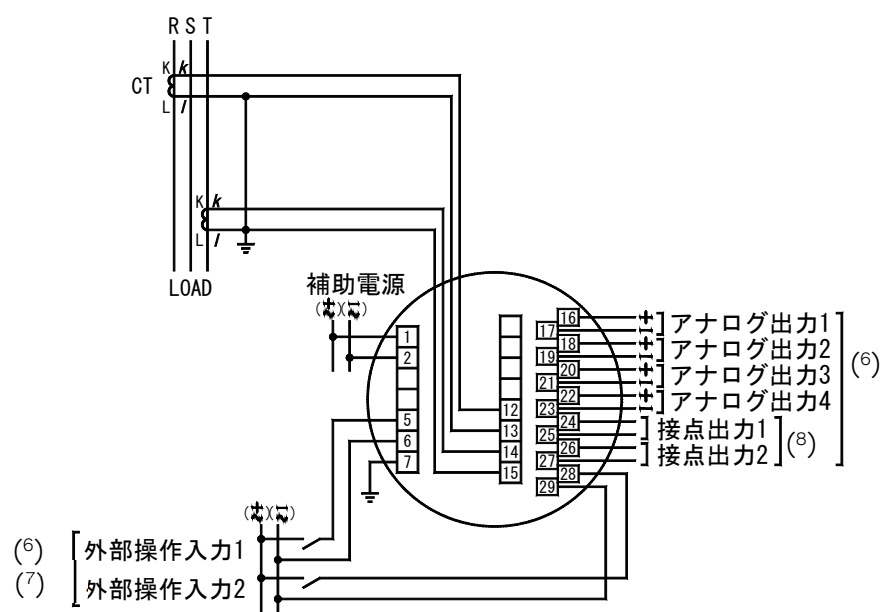
(14) 電流入力 3 \phi 3W (2CT)
