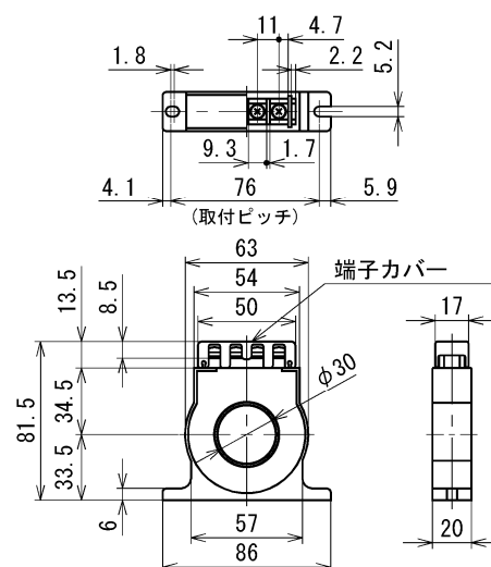
400A (OTG-LA68)
