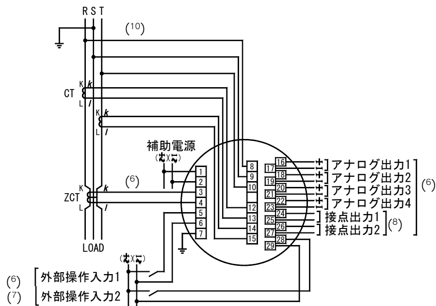
(3) 3 \phi 3W (S 相接地)
