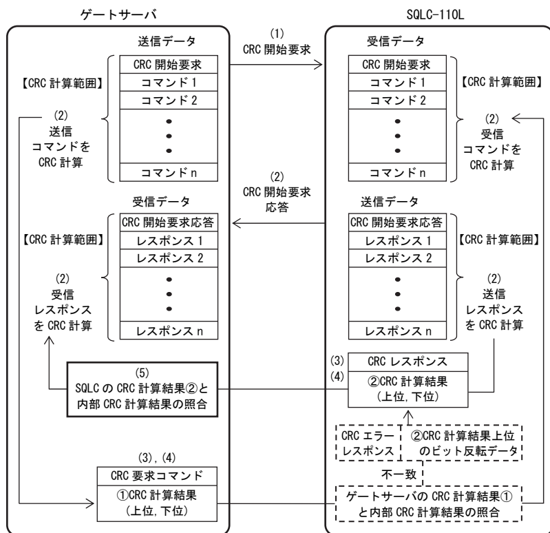
<CRC チェック概略図>
