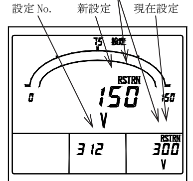
相電圧フルスケール (1φ3W)
