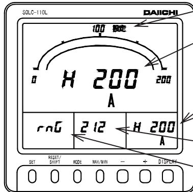
＜電流測定レンジ設定表示例＞
