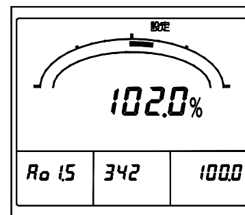
Ao1 スパン調整
