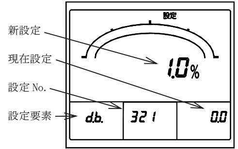
計測不感帯
