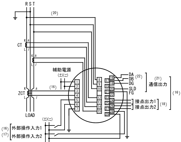
(3) 三相 3 線 (S 相接地)
