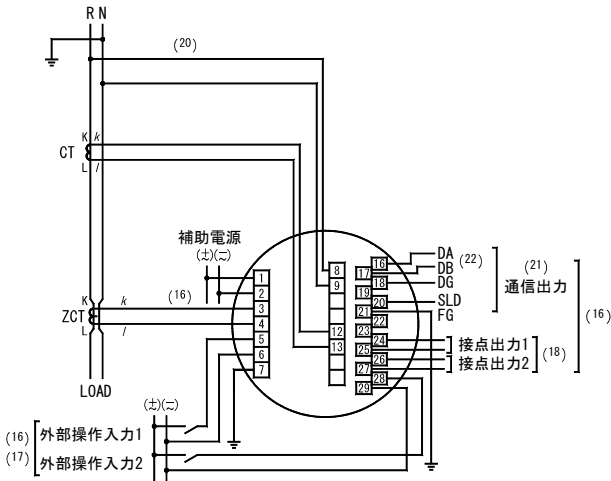
(1) 単相 2 線 (N 相接地)
