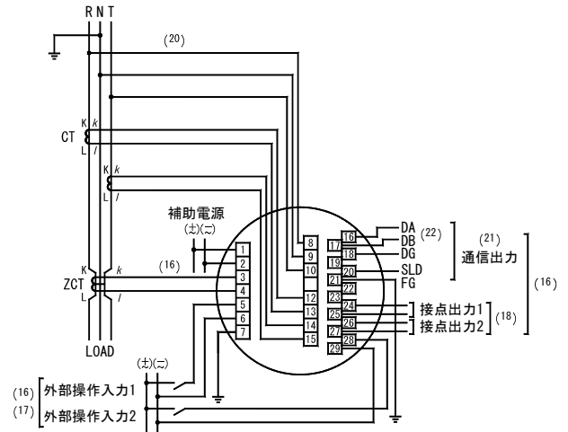
(2) 単相 3 線 (N 相接地)
