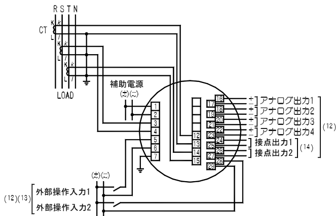
(3) 電流入力
