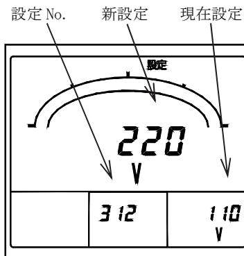
入力電圧
