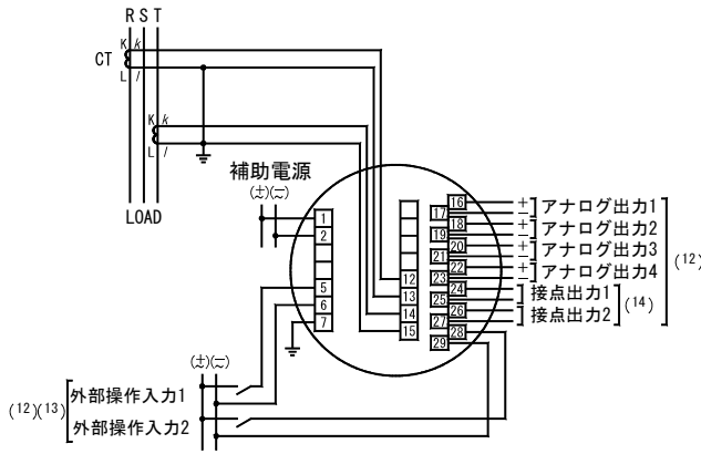
(5) 電流入力 3φ3W (2CT)
