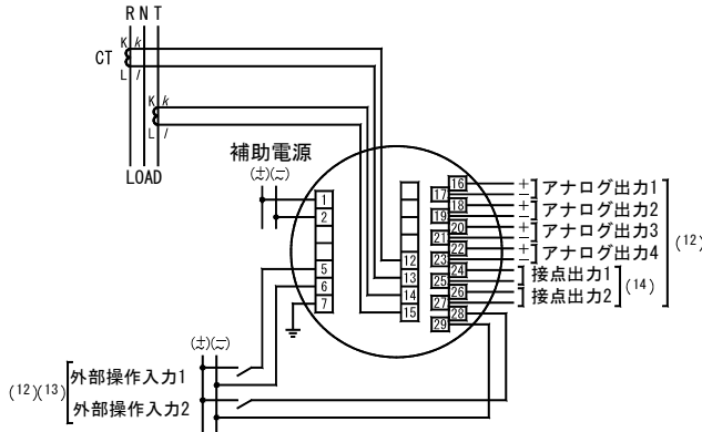
(7) 電流入力 1φ3W
