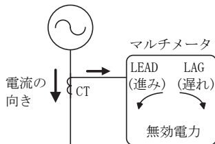
無効電力表示のイメージ図
