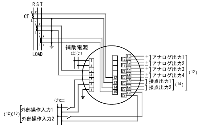
(6) 電流入力 3φ3W (3CT)
