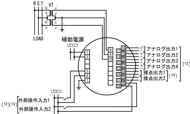
(9) 電圧入力 3φ3W
