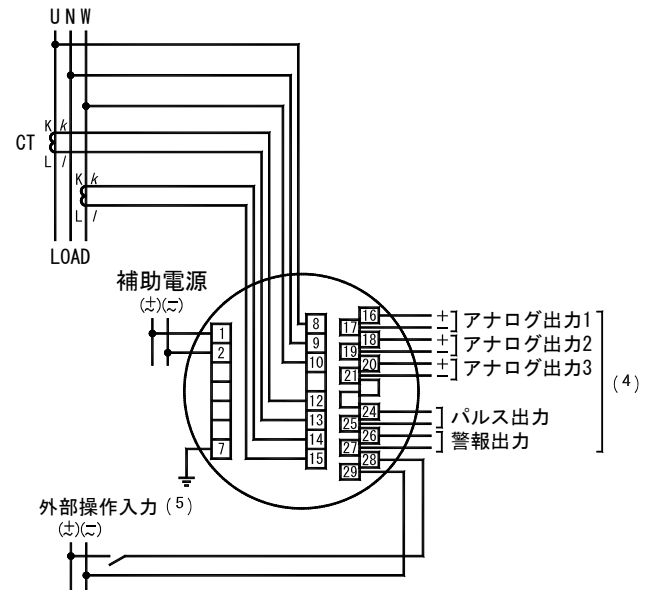
(2) 1φ3W, アナログ出力
