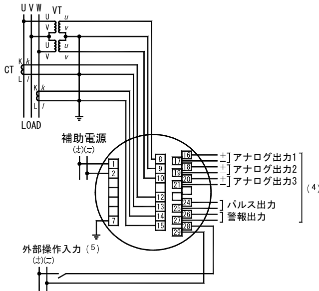
(3) 3φ3W, アナログ出力
