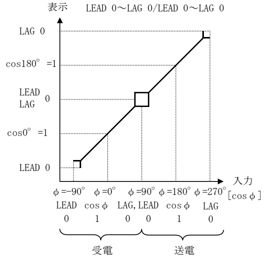
(潮流計測)
