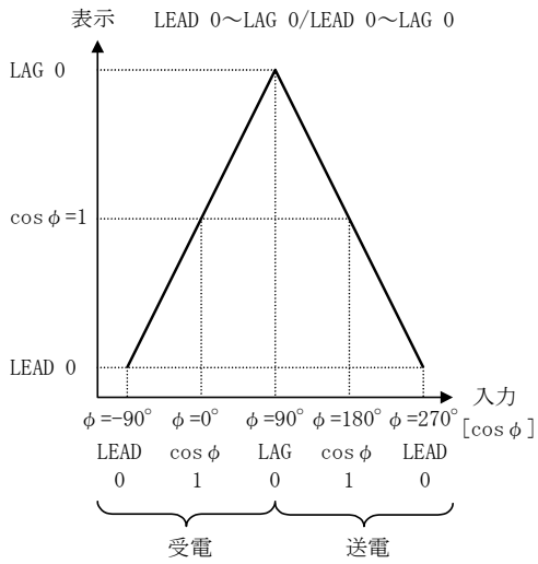
(一般計測)
