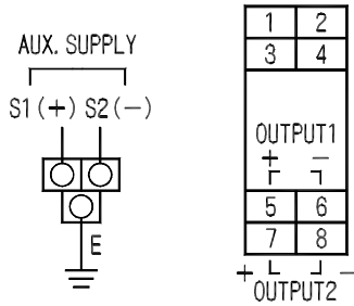
多連ベース (FWBA)
