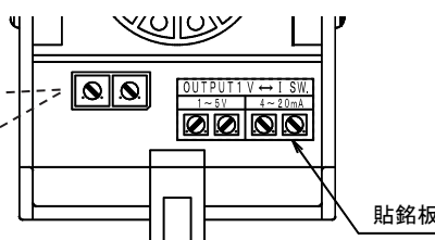
本体裏面図（ソケットを外した状態）
