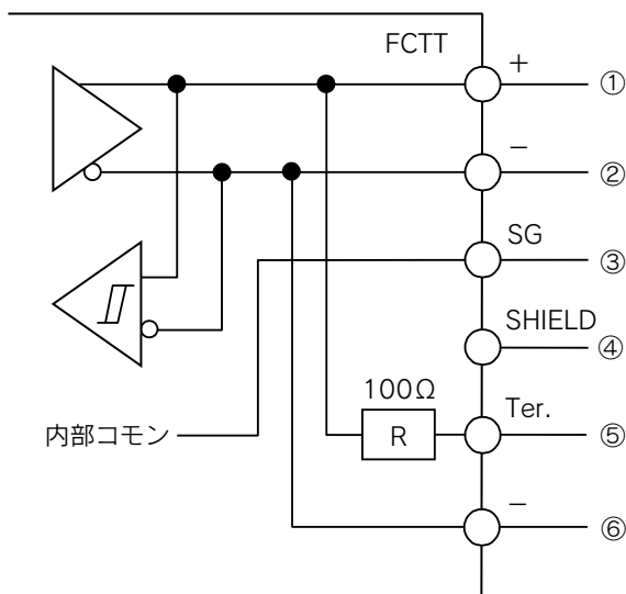
端子配列
