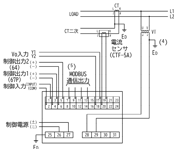
通信出力部の結線 (5)
