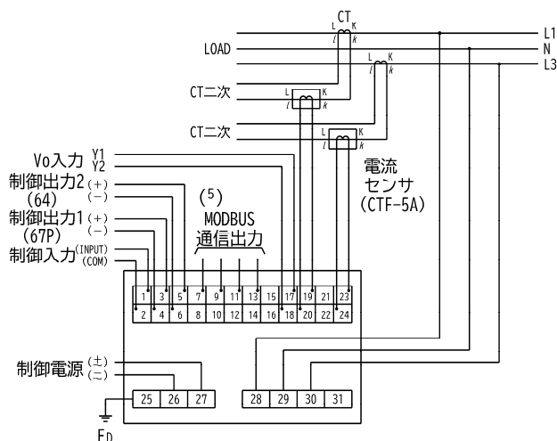
電流センサ接続図
