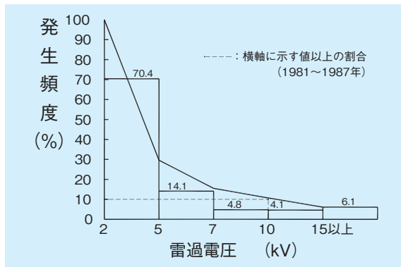
低圧配電線の雷過電圧の電圧別発生頻度
