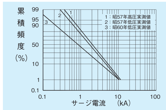
サージ電流実測値分布
