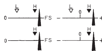
図2 片振れ計器
