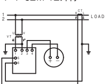
単相2線力率計 P T-62M-12外付
