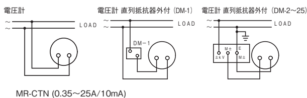
MR-CTN (0.35～25A/10mA)
