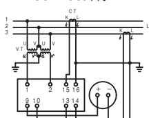
三相3線不平衡力率計 P T-63M-33外付
