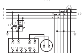
三相4線不平衡力率計 P T-64M-34外付
