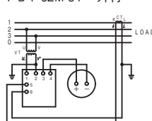
三相4線平衡力率計 P B T-62M-34 外付
