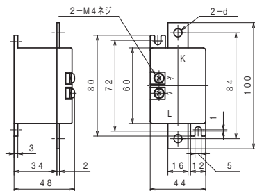
MR-CTN (30～100A/20mA)
