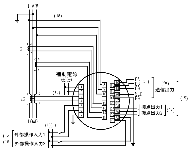
(3) 三相 3 線 (V 相接地)
